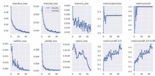
Fig.20 results for YOLO v5 epoch 50.
